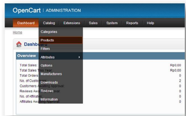
Gambar 16 Pengaturan Katalog
