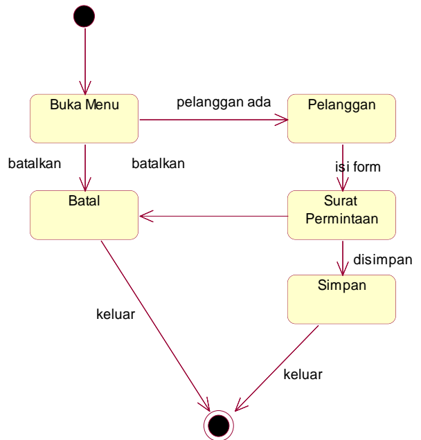
Sumber: Hasil Olahan Data Gambar 9 State chart Surat Permintaan
