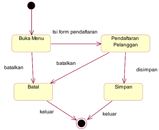
Sumber: Hasil Olahan Data Gambar 8 Statechart Data Pelanggan
