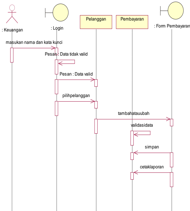
Sumber: Hasil Olahan Data Gambar 7 Sequence Diagram Pembayaran
