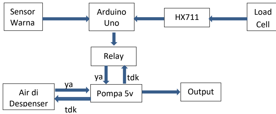
Gambar 7 Blok Diagram Rangkaian Sistem
