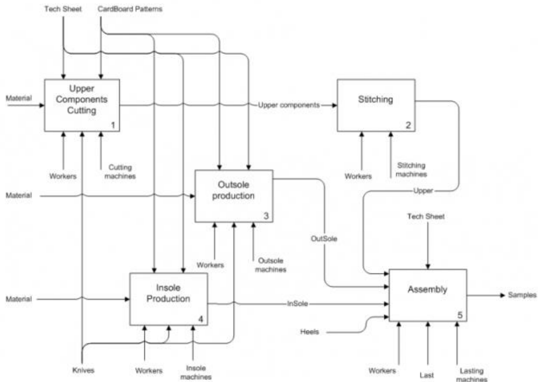
Gambar 3 Proses produksi sepatu
